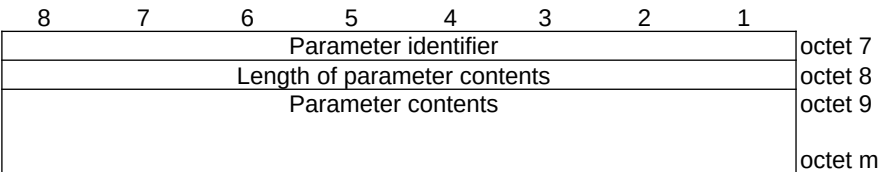
Figure 9.11.4.12.4: Parameter
