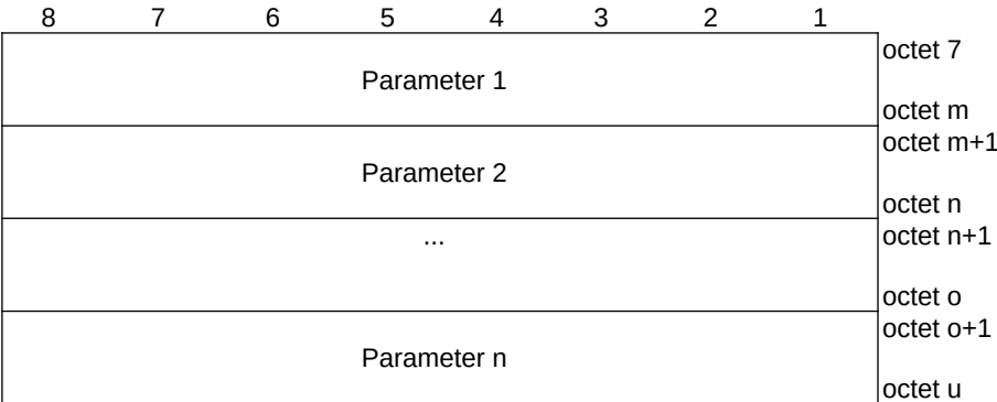
Figure 9.11.4.12.3: Parameters list
