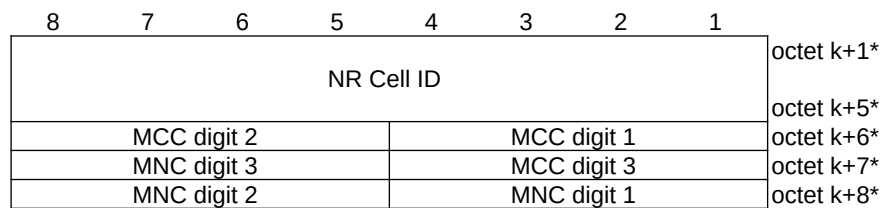
Figure 9.11.4.31.7: NR CGI
